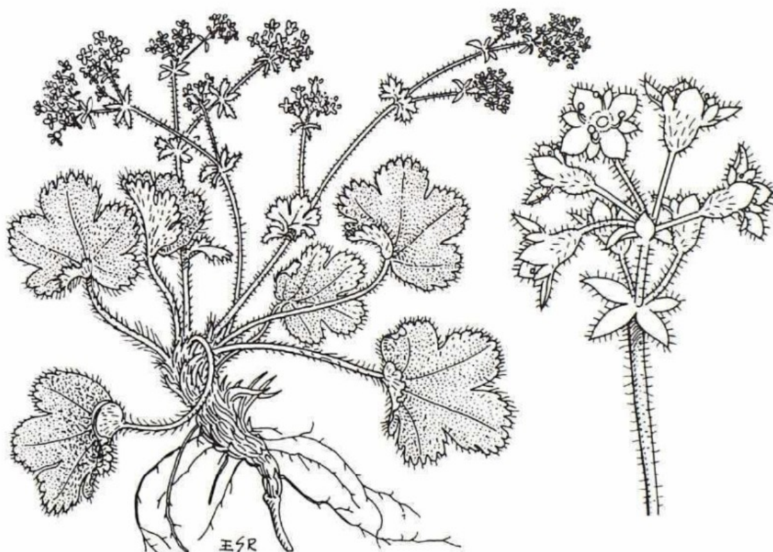
Alchemilla colorata . A la dreta, un fragment de la inflorescència (x 4).
