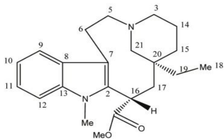
Vincaminorine (1)
