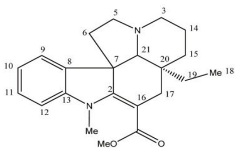
Minovine (3)
