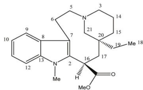
Vincaminoreine (2)
