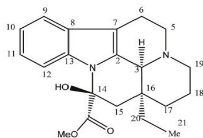
Vincamine (5)
